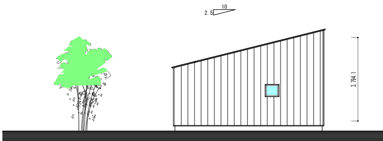
西立面図 S=1/100
