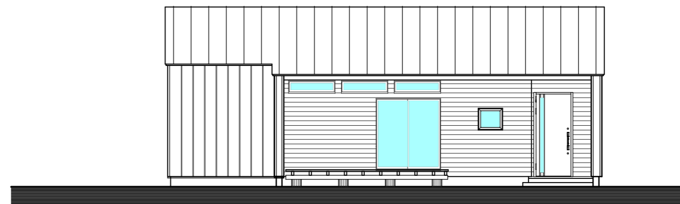
南立面図 S=1/100
