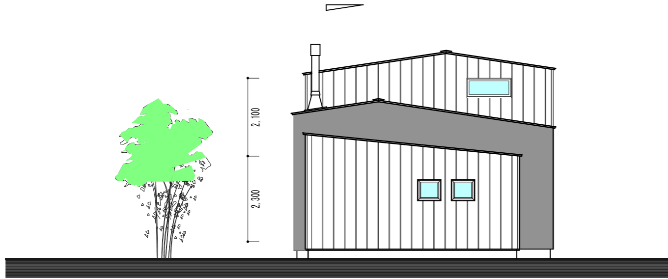
西立面图 S=1/100
