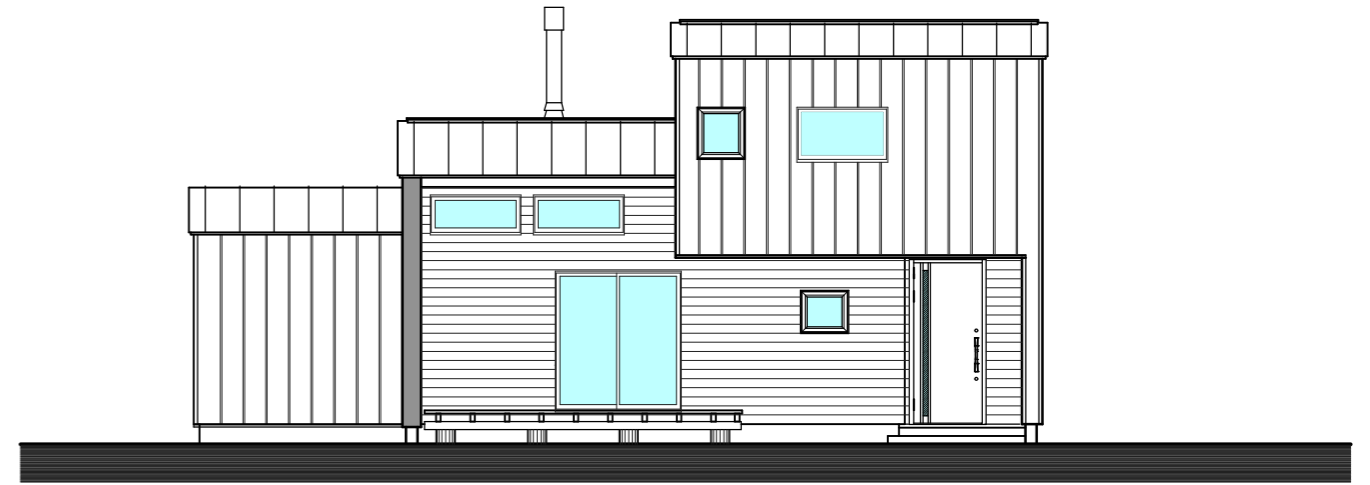
南立面图 S=1/100
