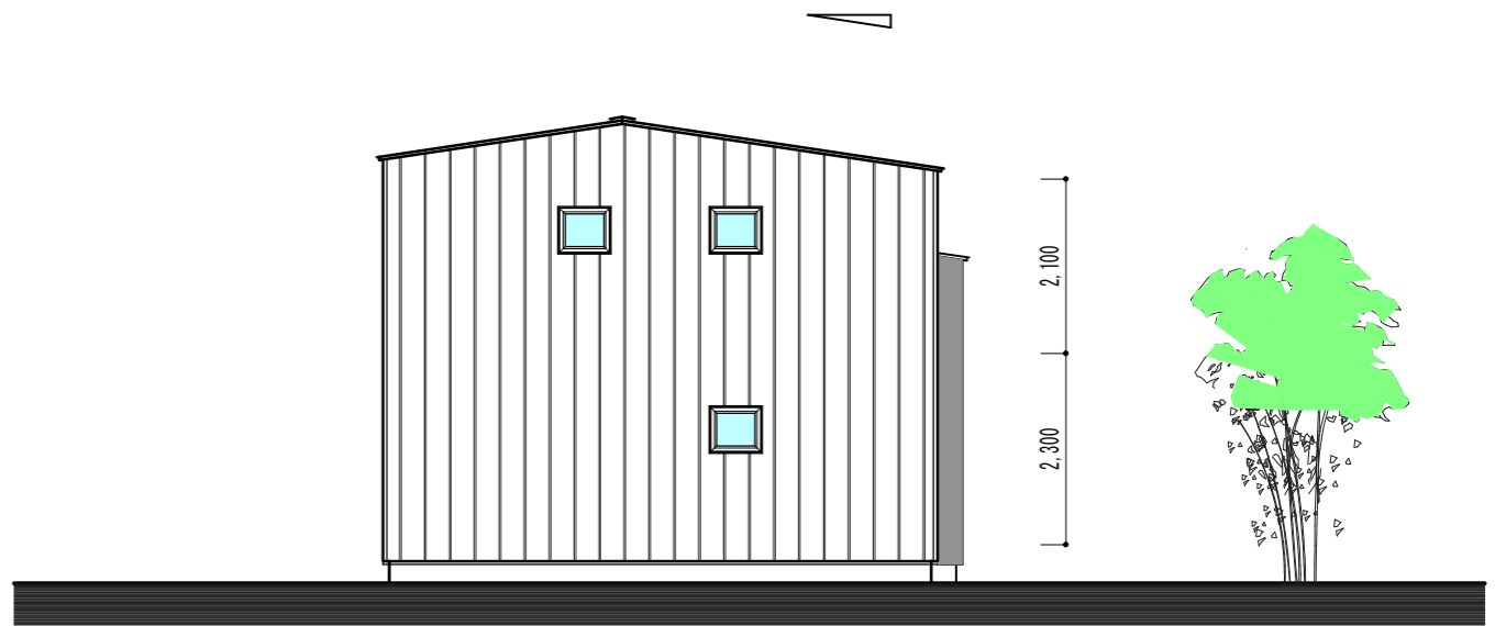
東立面图 S=1/100
