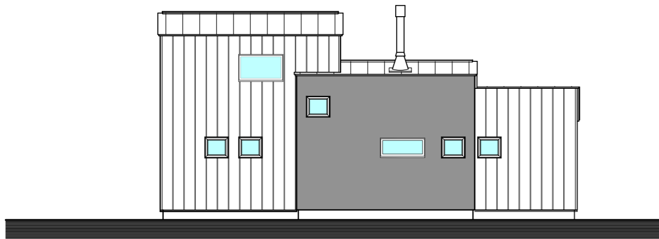
北立面图 S=1/100
