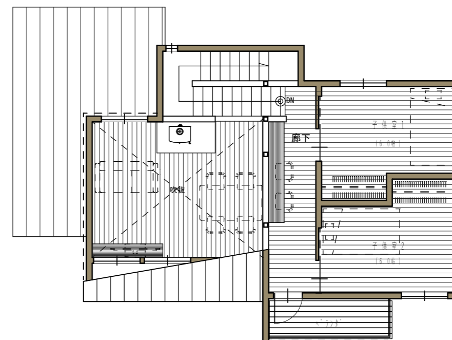
2 F-PLAN図 S=1/100
