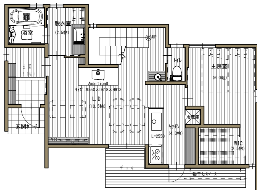
1 F-PLAN図 S=1/100
