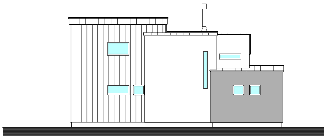
北立面图 S=1/100
